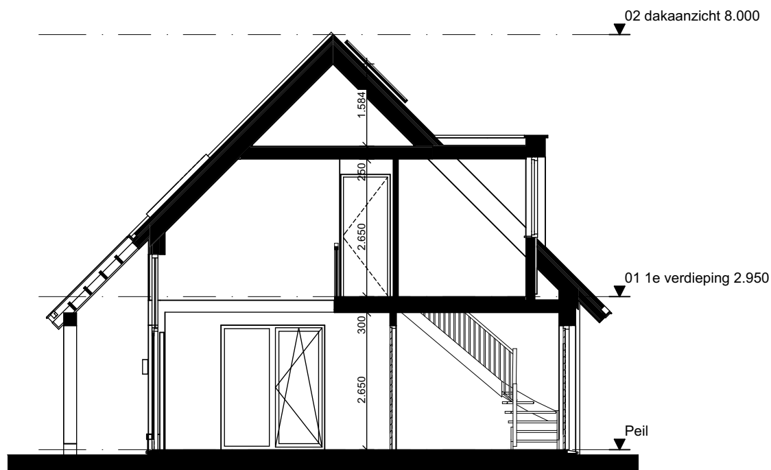
Doorsnede A-A - 1:100
