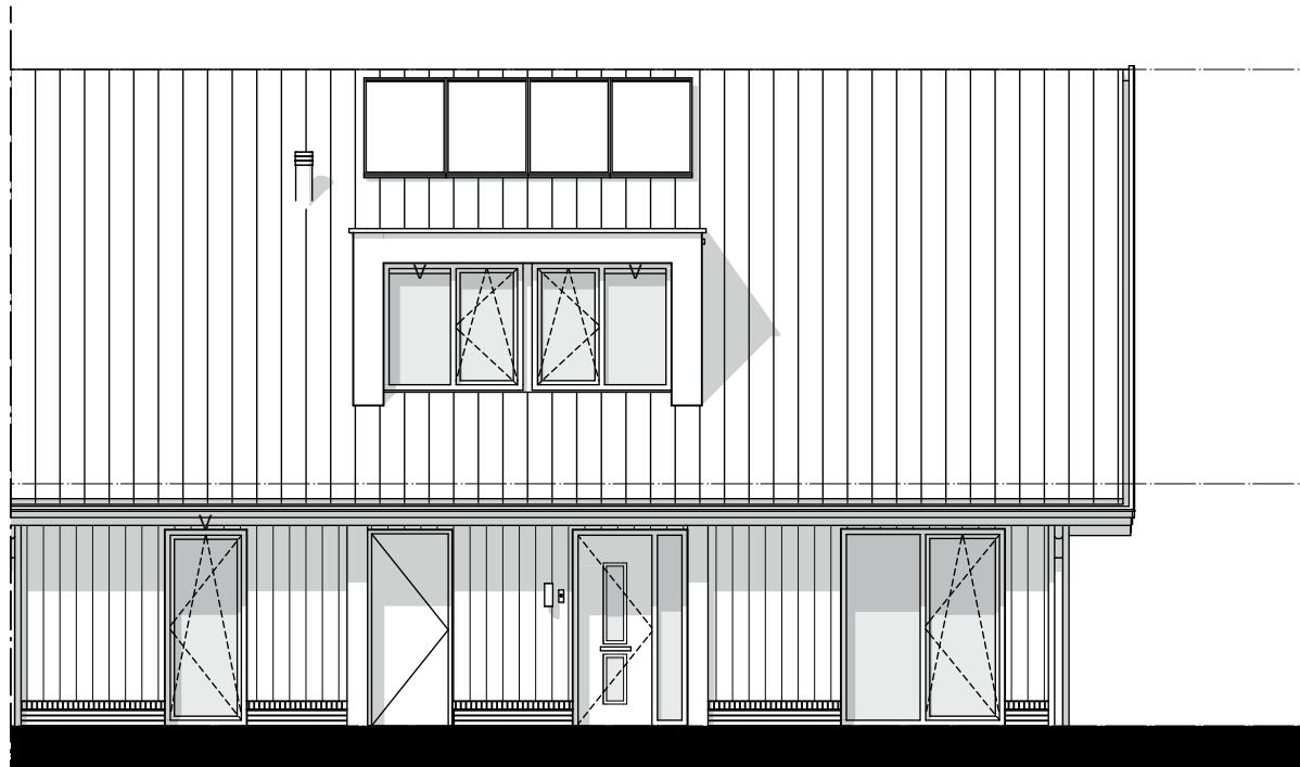
Vorgevel - 1:100
