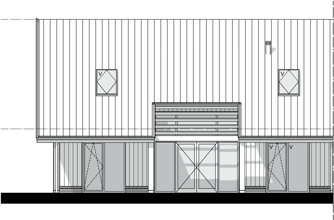
Achtergevel - 1:100
