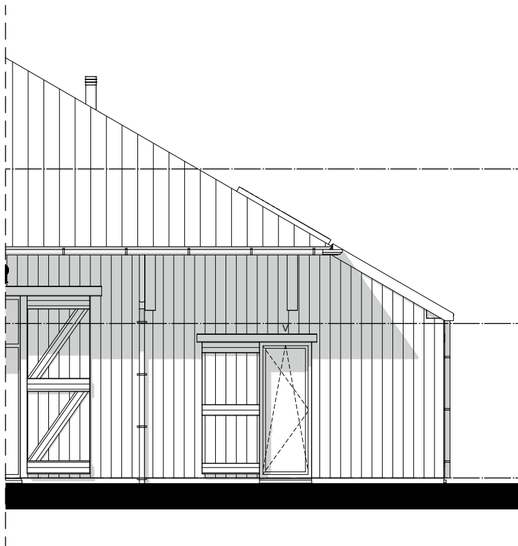
Zijgevel - 1:100
