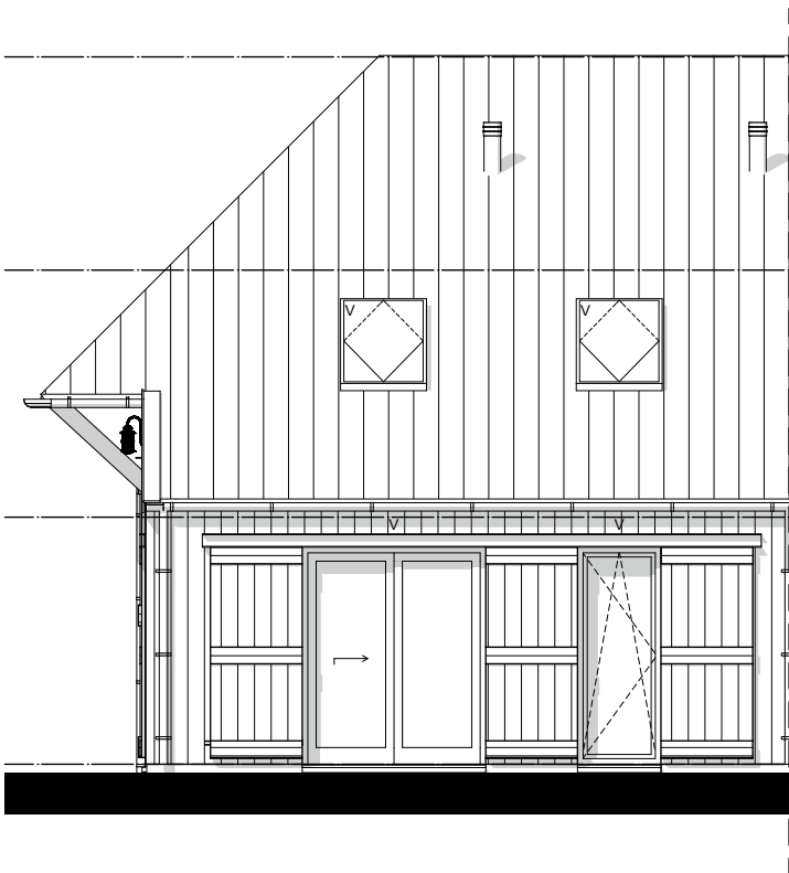
Voorgevel - 1:100
