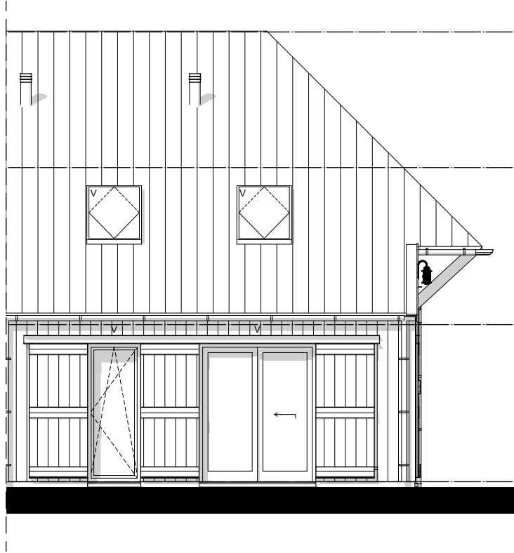
Vorgevel - 1:100
