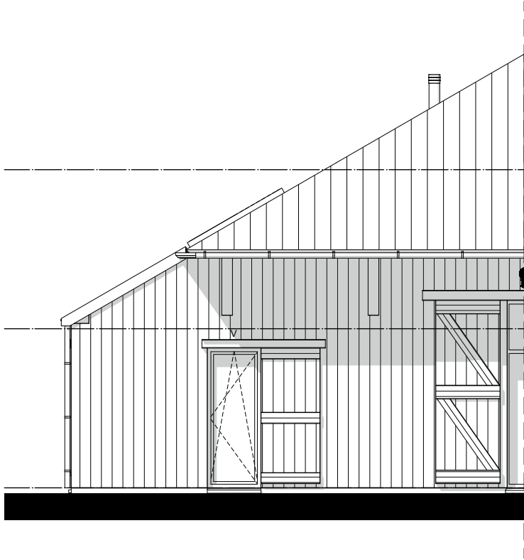
Zijgevel - 1:100
