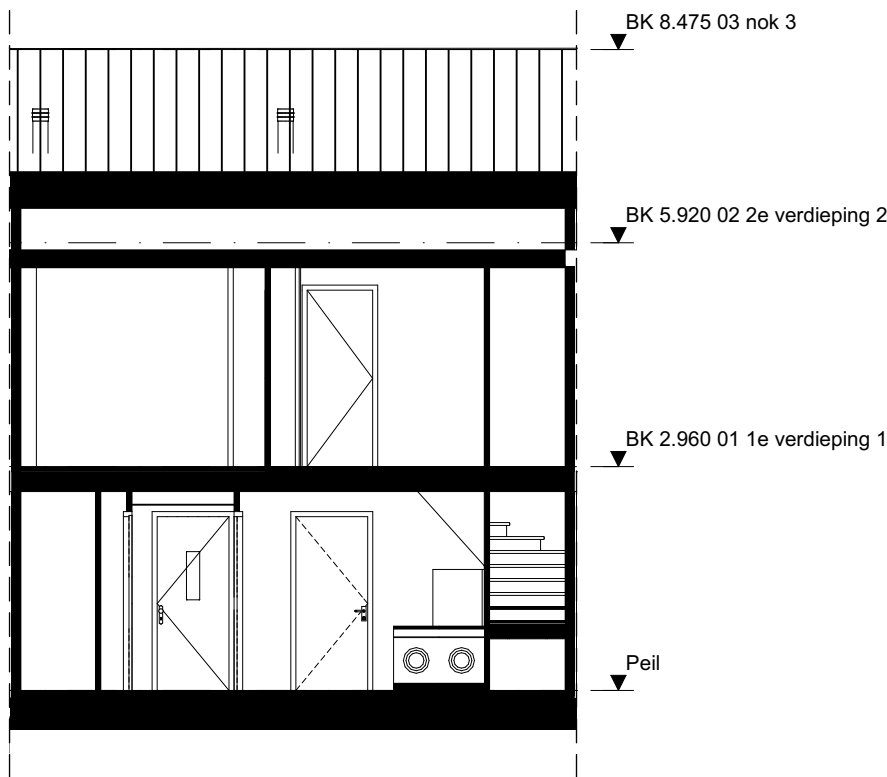
Doorsnede B-B - 1:100
