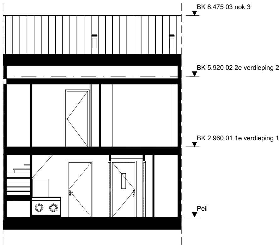
Doorsnede B-B - 1:100
