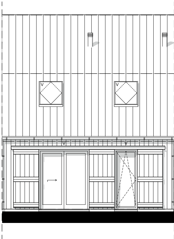
Voorgevel - 1:100
