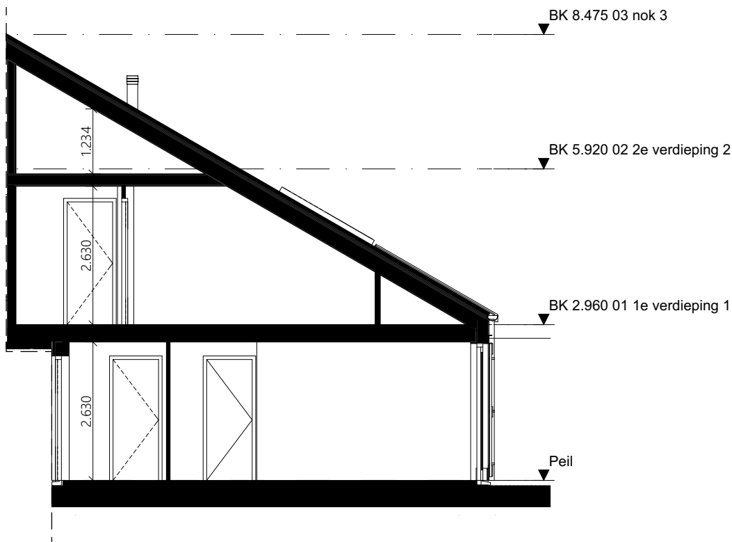
Doorsnede A-A - 1:100
