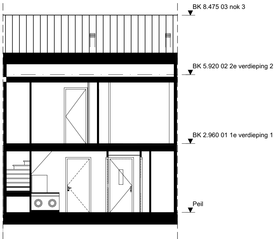
Doorsnede B-B - 1:100
