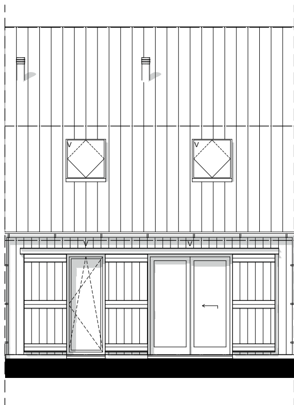
Voorgevel - 1:100
