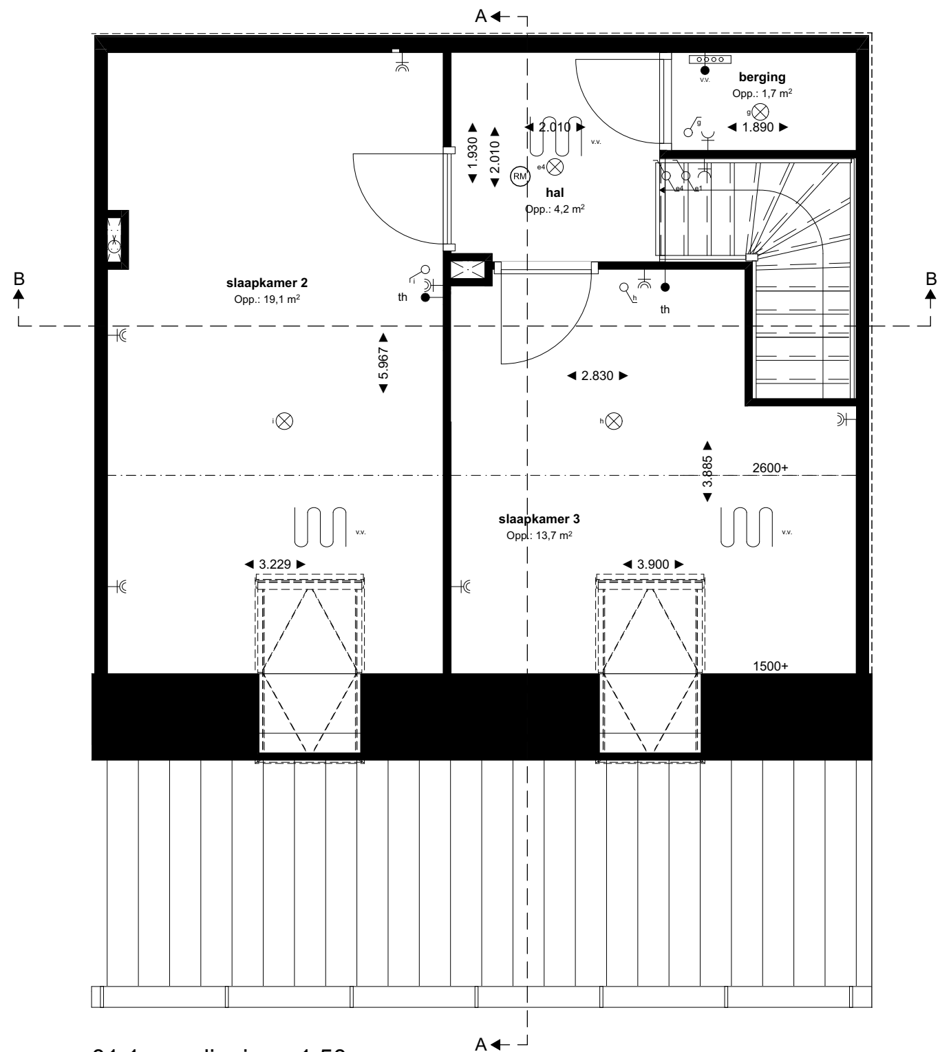
01 1e verdieping - 1:50
