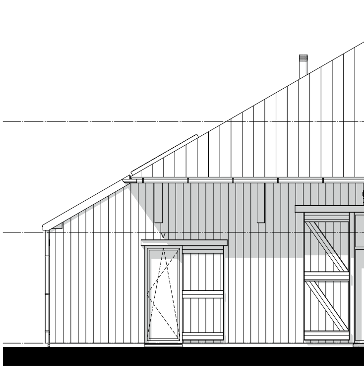
Zijgevel - 1:100
