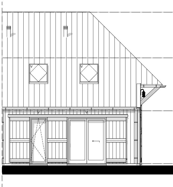
Voorgevel - 1:100
