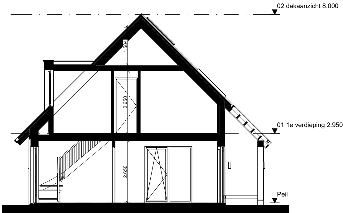
Doorsnede A-A - 1:100
