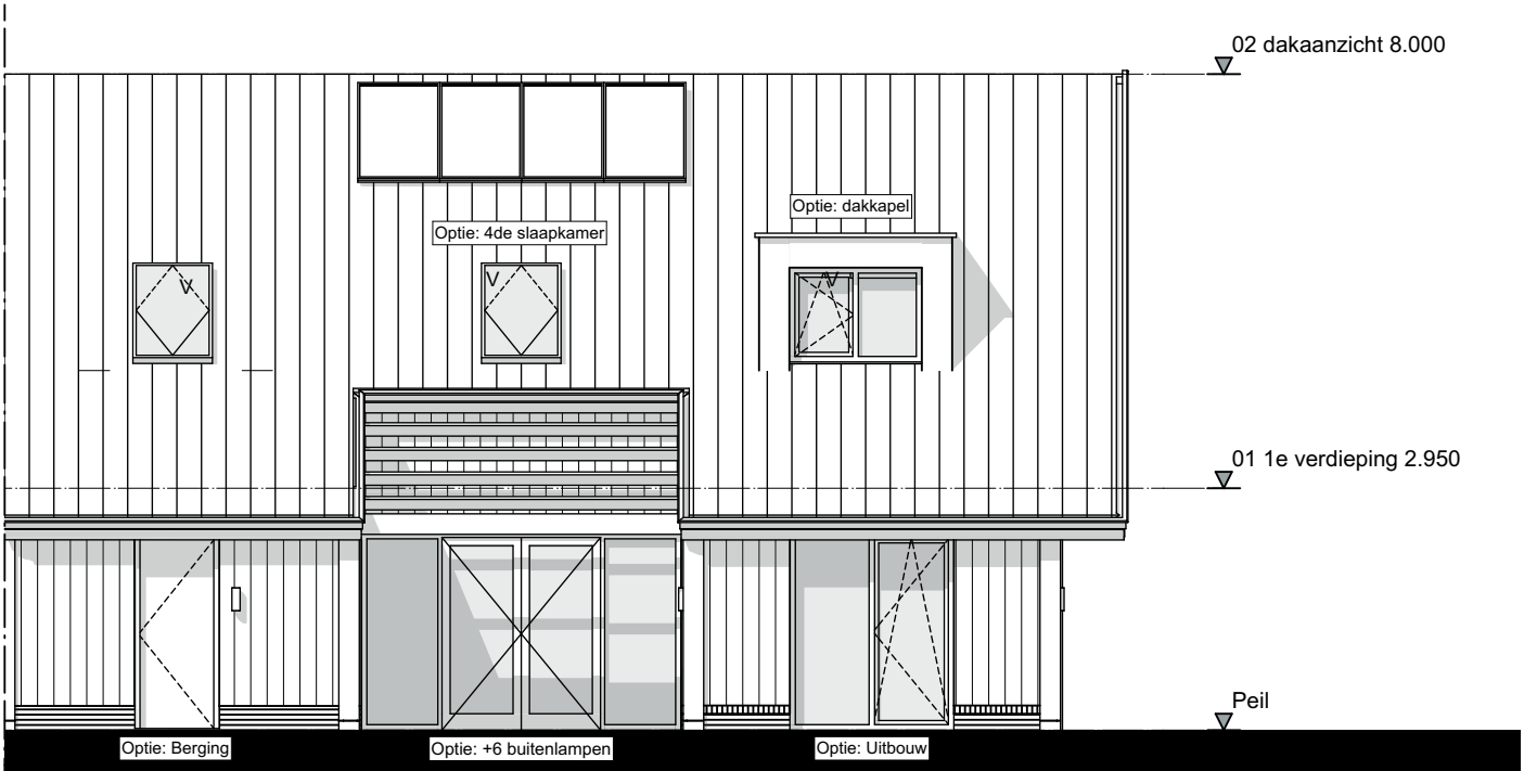
Achtergevel - 1:100
