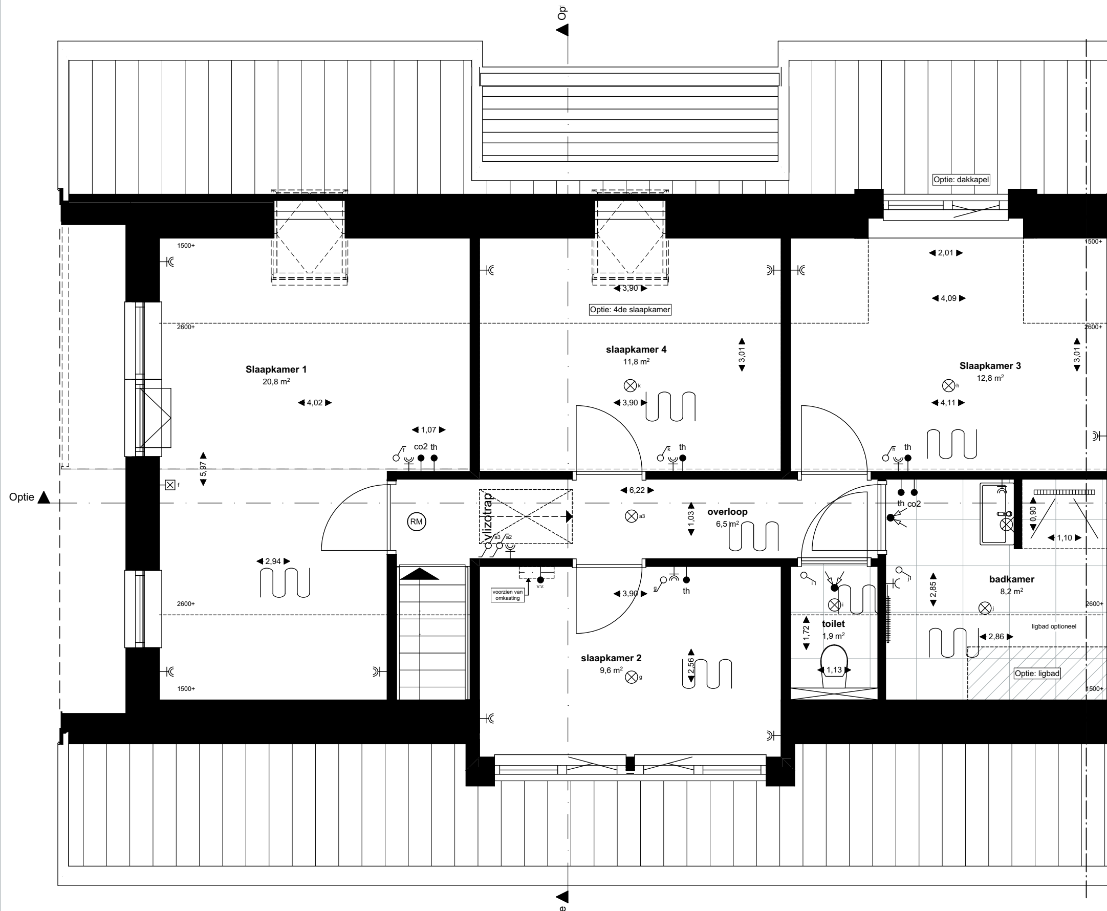
01 1e verdieping - 1:50
