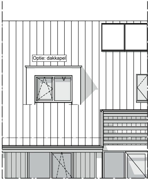
Achtergevel - 1:100
